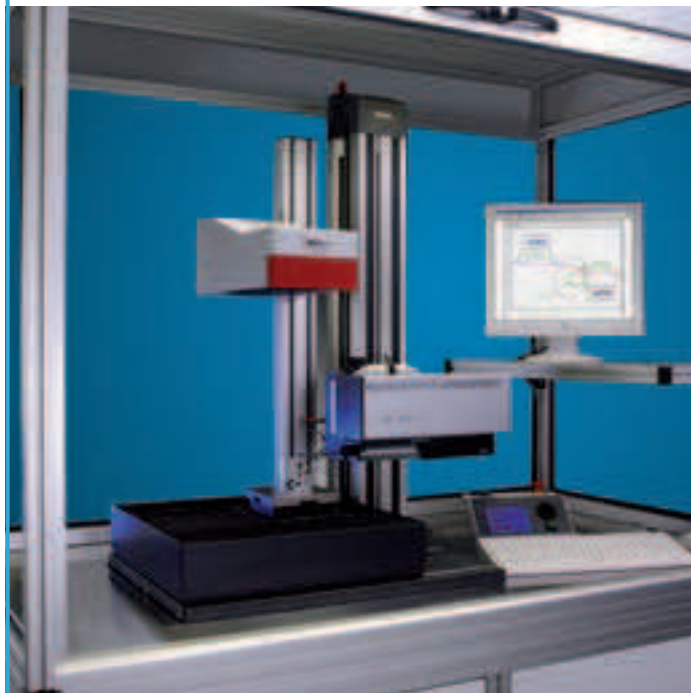
MarSurf LD 130 с устройством автоматической смены щупов консолей TWE
